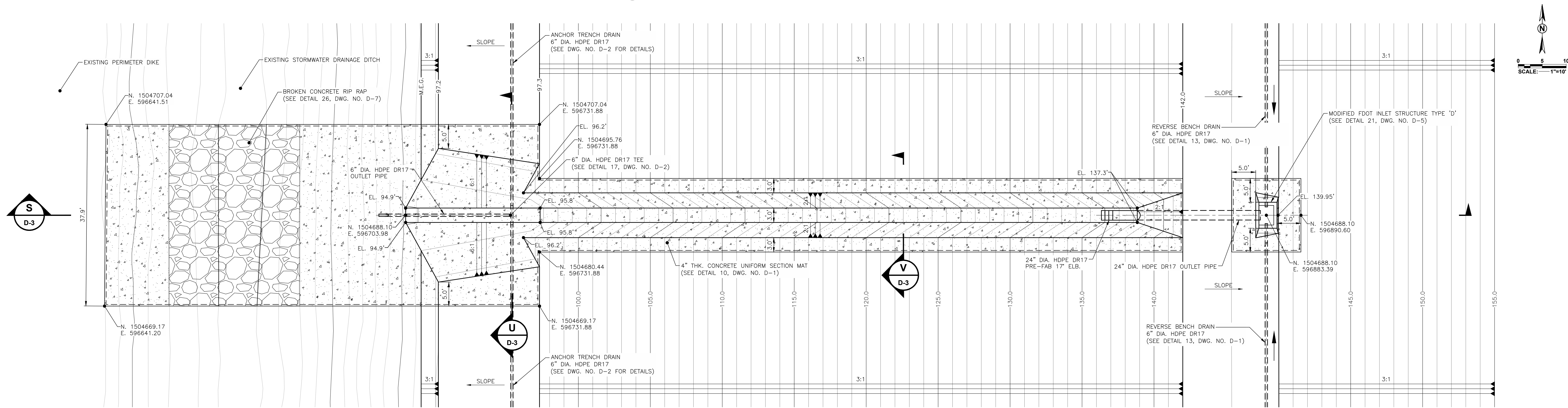
4 CONCRETE FLUME NO. 2 PLAN VIEW SCALE: 1" = 10' G-12 CS-1 CS-2 CS-3 CS-4
