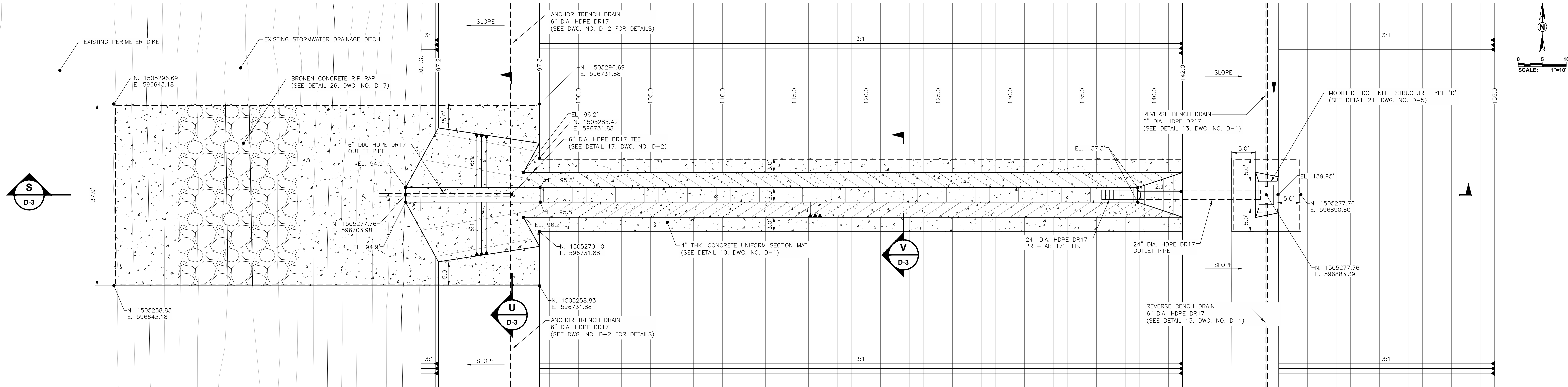
3 CONCRETE FLUME NO. 1 PLAN VIEW SCALE: 1" = 10' G-12 CS-1 CS-2 CS-3 CS-4
