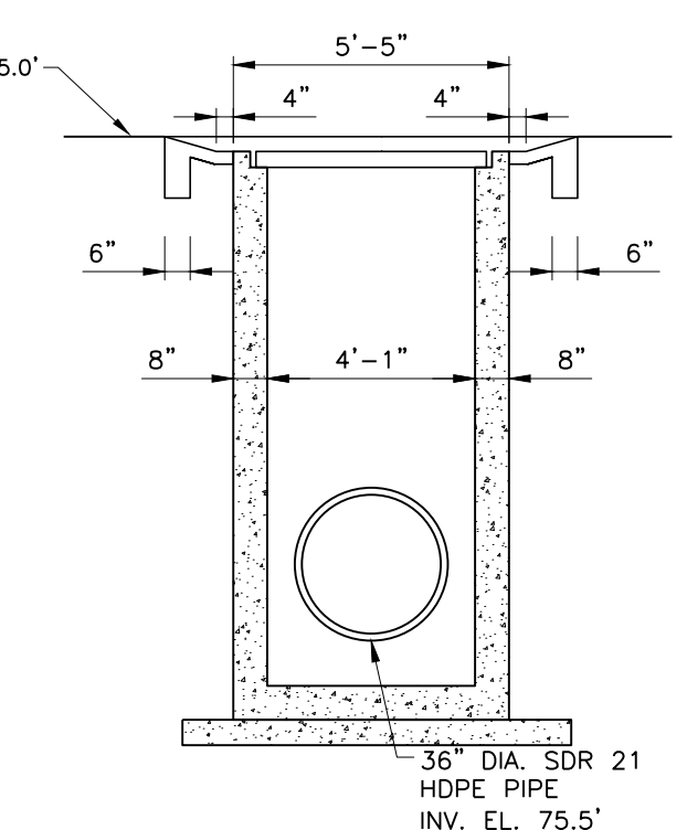
SCALE: 1" = 50'
